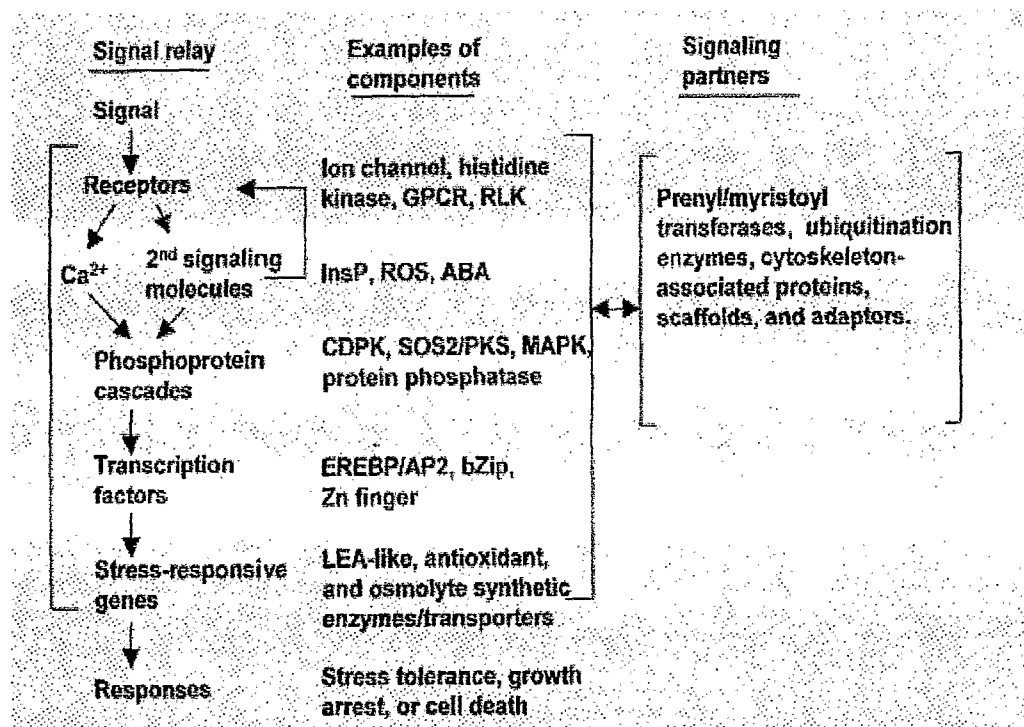
تصویر ۲: مسیر رایج انتقال پیام تنش های سرما، خشکی و شوری در گیاهان (Xiong et al., 2002).
